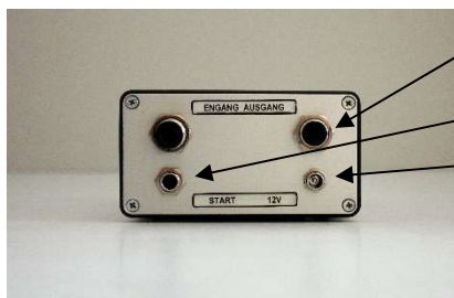
Bild 2 - Rückseite SDT-DG-1
