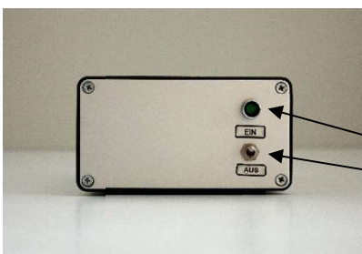
Bild 3 - Frontseite SDT-DG-1
